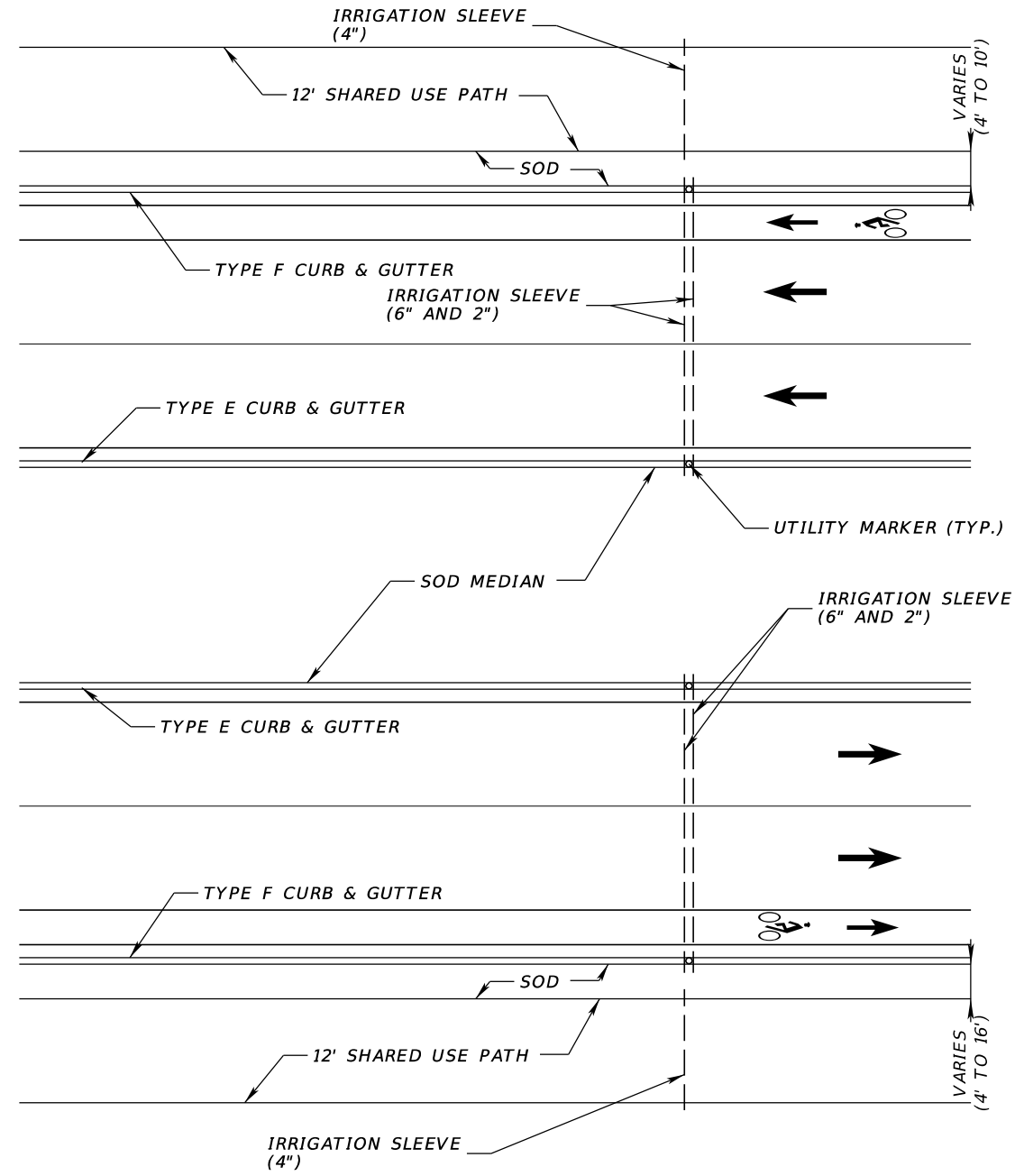
IRRIGATION SLEEVE DETAILS N.T.S.
