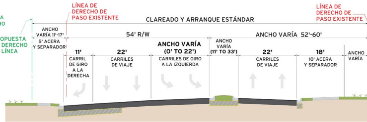
SECCION TÍPICA | FORTUNE ROAD
