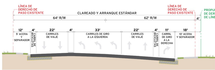
SECCION TÍPICA | FORTUNE ROAD
