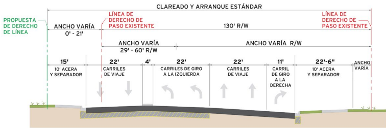
SECCION TÍPICA | SIMPSON ROAD
